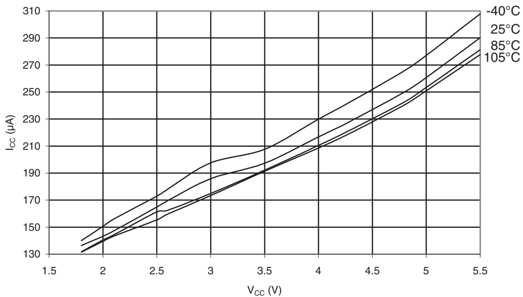
Figure 31-87. ATmega48PA: ADC Current vs. V CC (AREF = AV CC )
