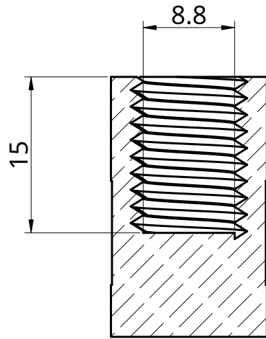
A - A
