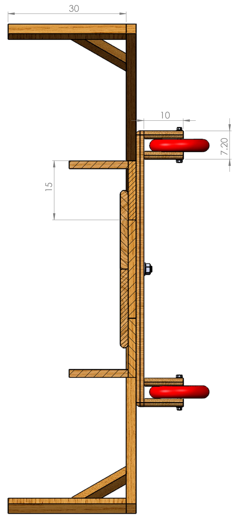
SECTION A-A SCALE 1 : 5
