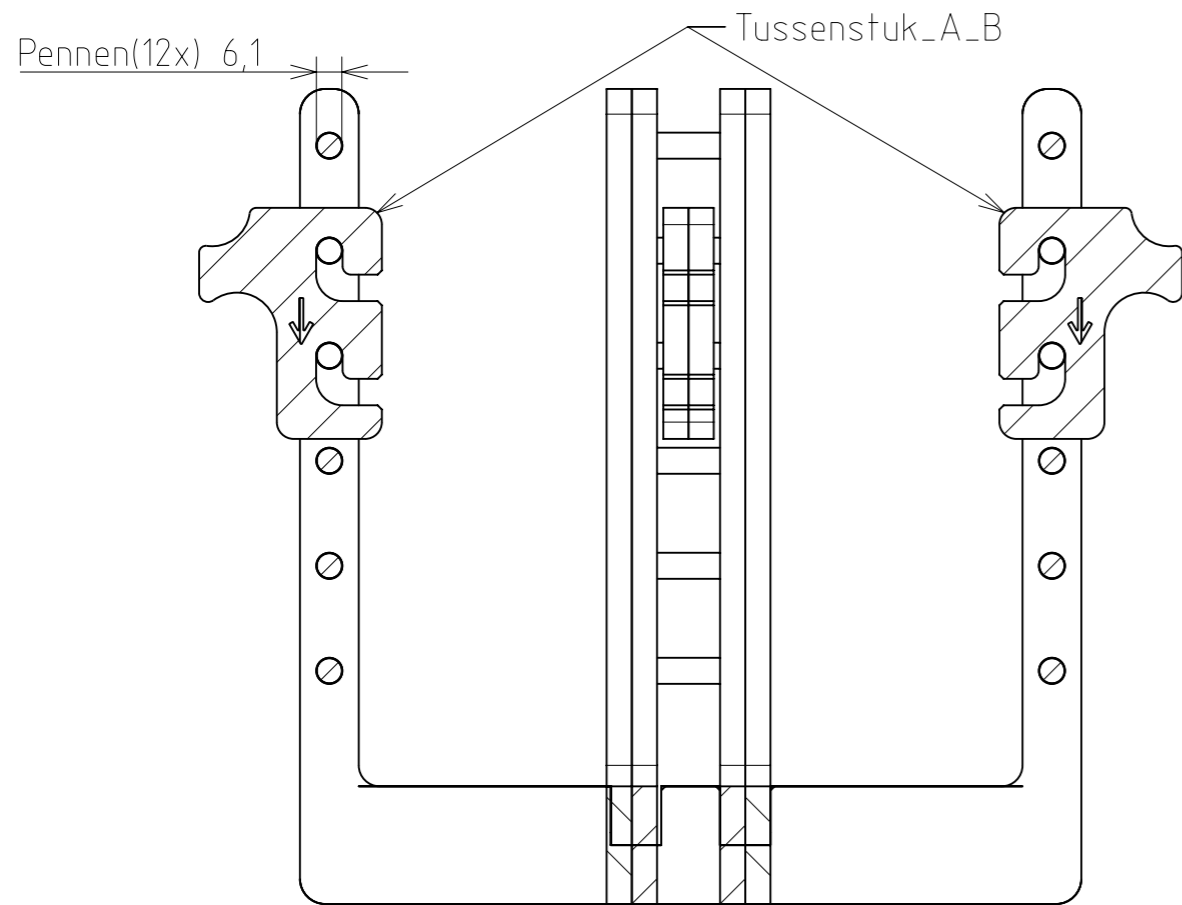
SECTION A-A
